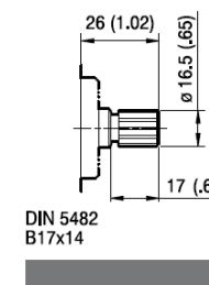
T2 Coppia Max Max Torque 130 Nm
