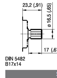
T1 Coppia Max Max Torque 130 Nm
