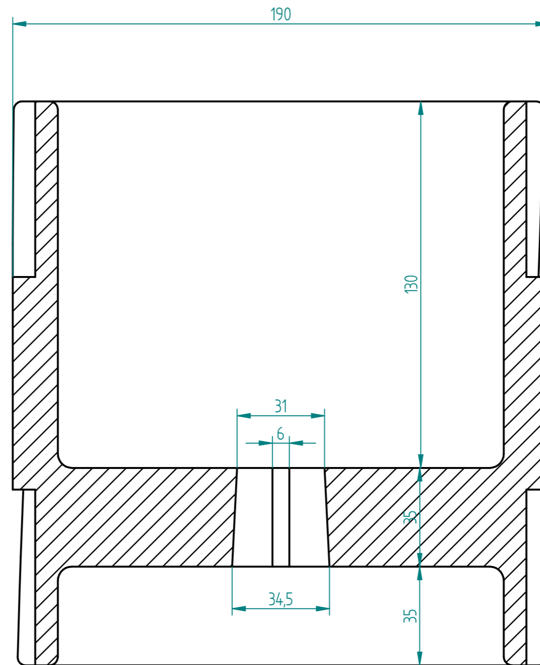
SECTION A-A
